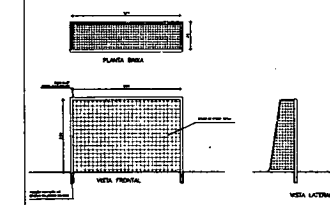
05 DET. BALSA FÚTEBO ESCALA = 1/30
