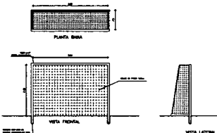
01 DET. BALISA FUTEBOL ESCALA = 1:50
