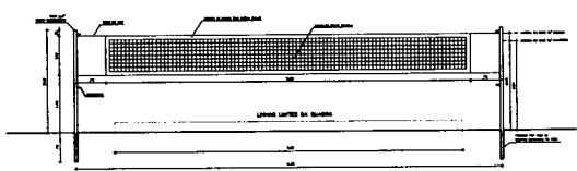
01 DET. REDE DE VOLEY ESCALA = 1:50
