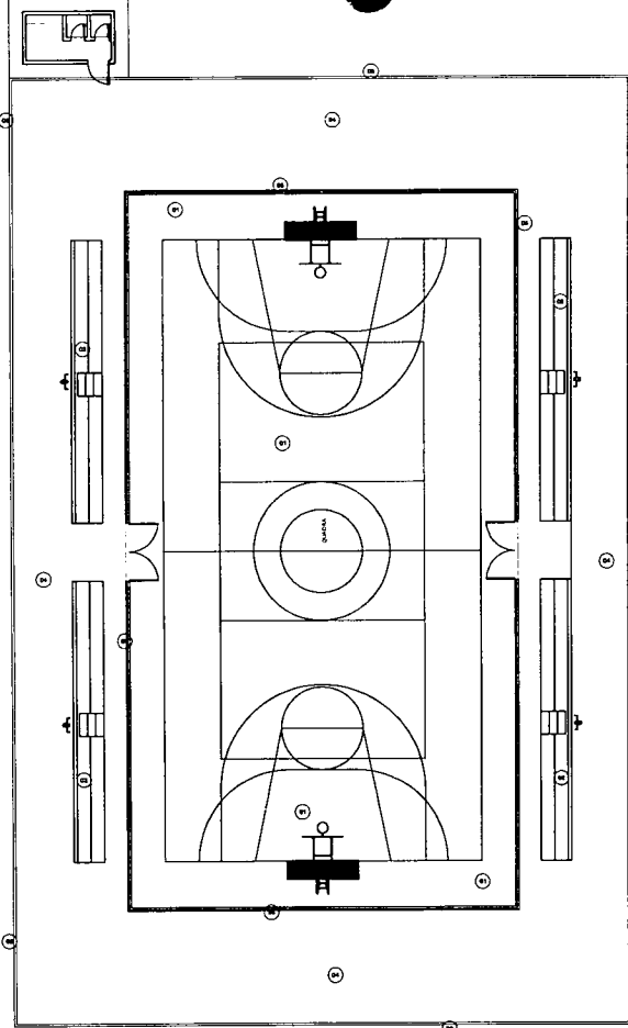
01 DIAGRAMA DE PISO ESCALA = 1:125
