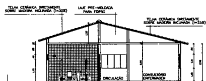
CORTE AA ESCALA 1:100
