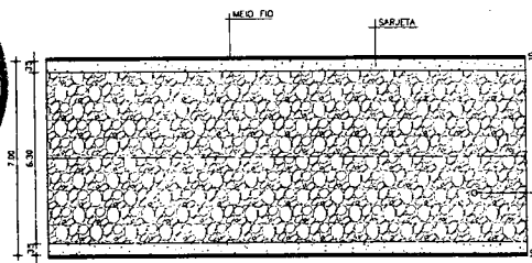
06 DETALHES DA VIA ESCALA - 1:75
