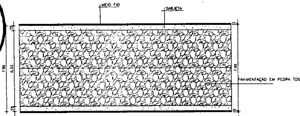
06 DETALHES DA VIA ESCALA - 1:75
