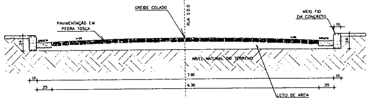
04 SEÇÃO TRANSVERSAL/DET. CONSTRUTIVO ESCALA = 1:25
