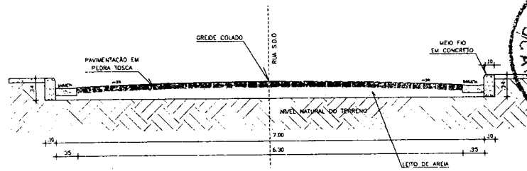
04 SEÇÃO TRANSVERSAL/DET. CONSTRUTIVO ESCALA - 1:25
