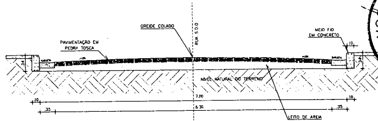
04 SEÇÃO TRANSVERSAL/DET. CONSTRUTIVO ESCALA - 1:25
