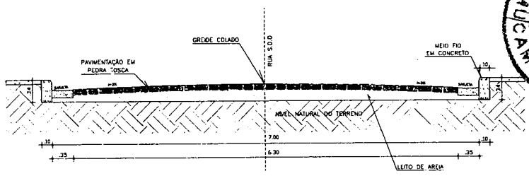
04 SEÇÃO TRANSVERSAL/DET. CONSTRUTIVO ESCALA - 1:25
