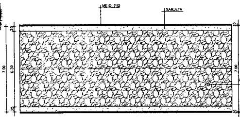
06 DETALHES DA VIA ESCALA - 1:75
