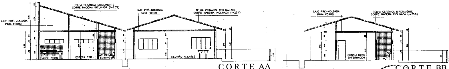
CORTE AA
