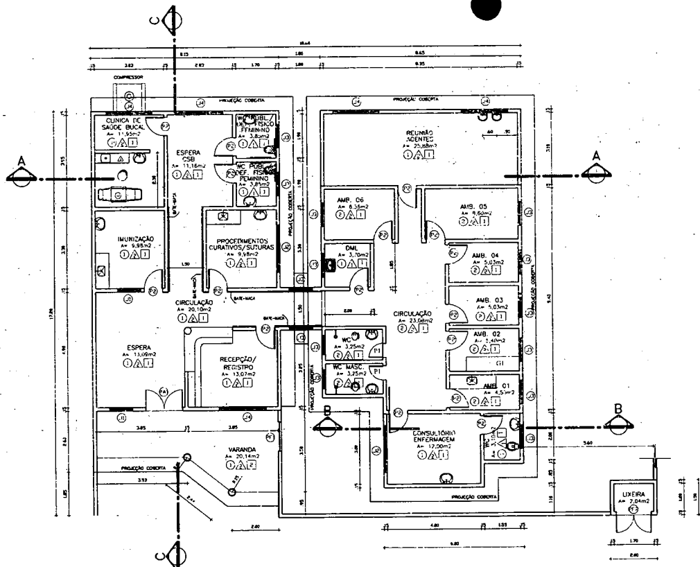
PLANTA BAIXA - OBRA
