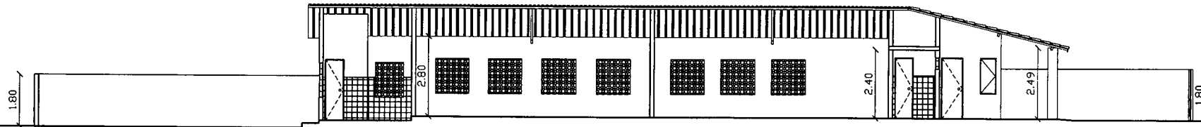
01 CORTE A - A ESCALA - 1:125
