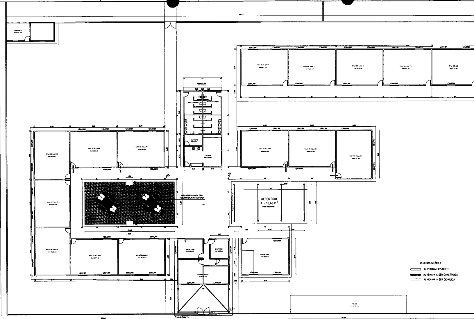
01 PLANTA BAIXA EXECUTIVA ESCALA - 1:125
