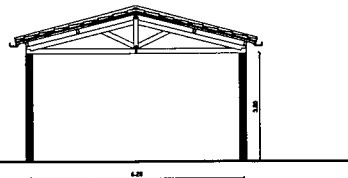
02 DE. COBERTA DO REFEITÓRIO ESCALA - 1:75
