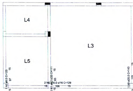
2 ARMAÇÃO NEGATIVA DAS LAJES DO PAVIMENTO TÉRREO ESCALA 1:50
