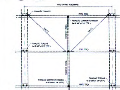
4 MONTAGEM DOS TIRANTES E CORRENTE RÍGIDAS ESCALA 1/10
