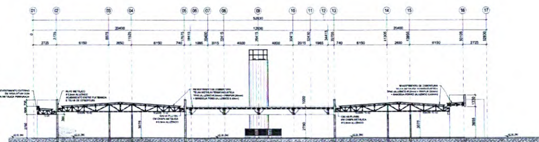
3 ELEVÇÃO TRANSVERSAL - EIXO "F" ESCALA 1/100
