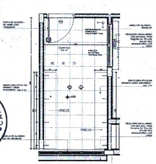
PLANTA BAIXA
