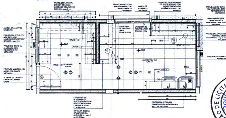
PLANTA BAIXA
