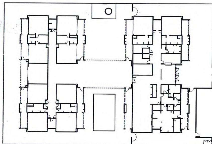
2 PLANTA BAIXA ESCALA: 1/200
