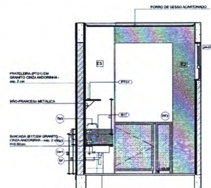
VISTA 04
