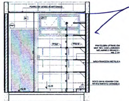
VISTA 02
