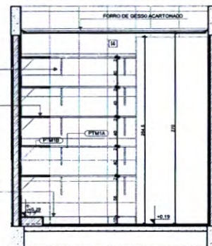
VISTA 03
