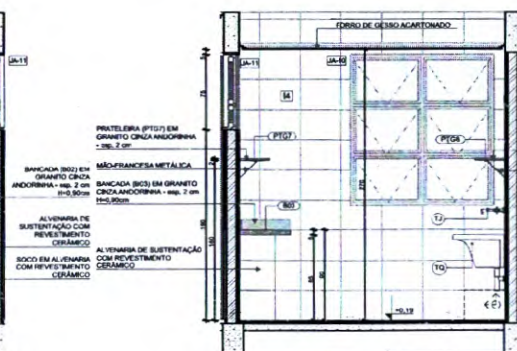
VISTA 05
