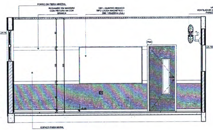
VISTA 02
