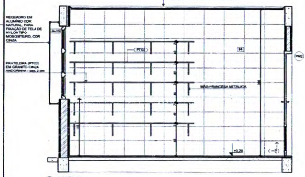
VISTA 02
