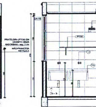
VISTA 06
