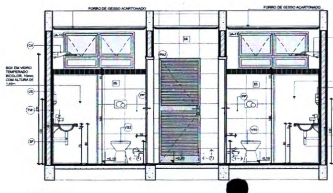
VISTA 02
