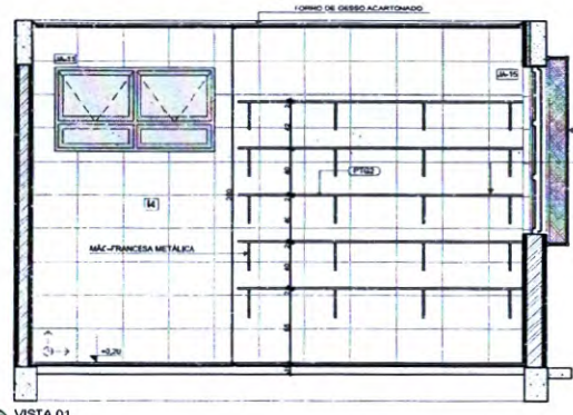
VISTA 01
