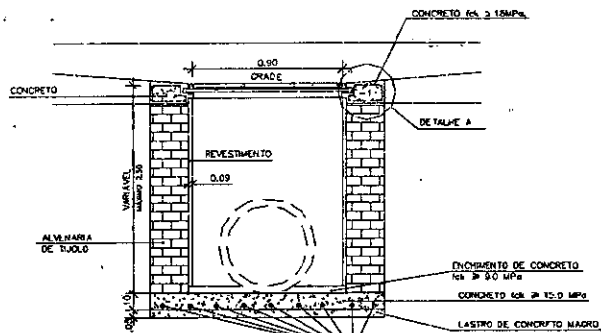
CORTE - AA
