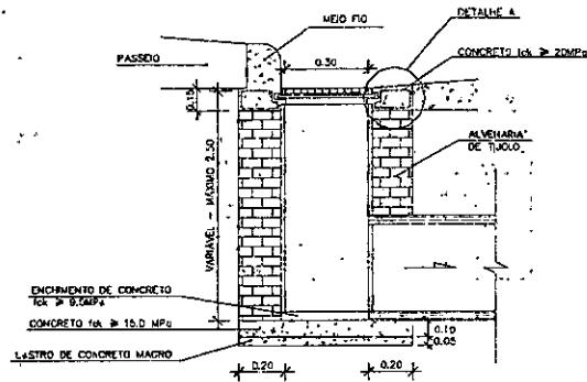
CORTE - BB
