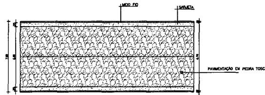
06 DETALHES DA VIA ESCALA - 1/75
