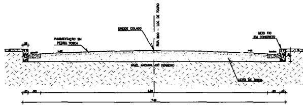
05 SEÇÃO TRANSVERSAL/DET. CONSTRUTIVO ESCALA - 1/25
