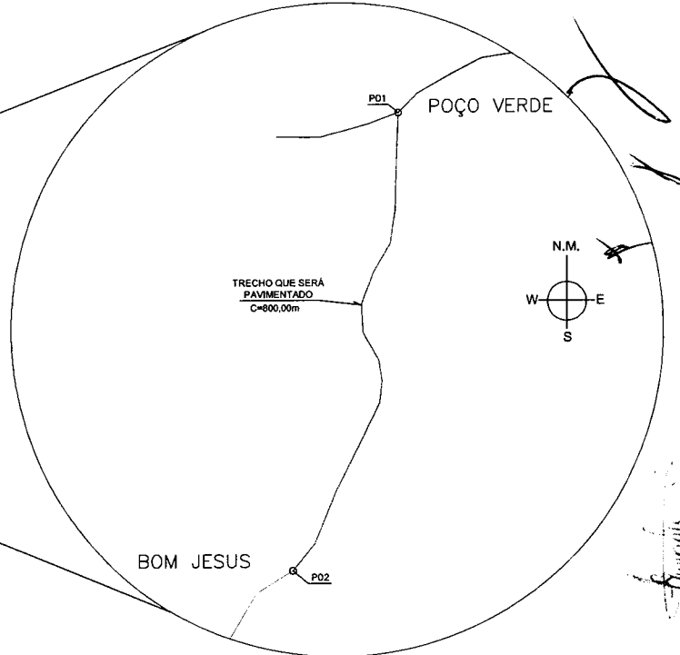
02 ARRUAMENTO ESCALA - 1:1200
