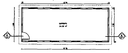
01 PLANTA BAIXA ESCALA = 1/75
