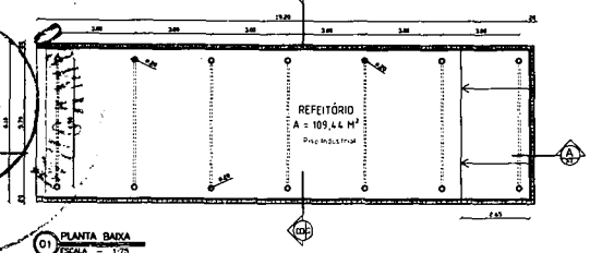
01 PLANTA BAIXA ESCALA = 1/75
