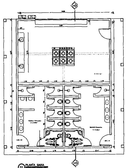
01 PLANTA BAIXA ESCALA = 1/50
