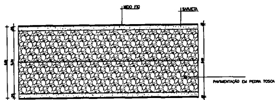
06 DETALHES DA VIA ESCALA - 1:75
