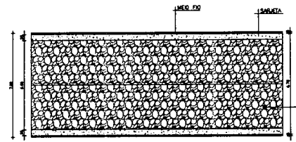
06 DETALHES DA VIA ESCALA - 1:75
