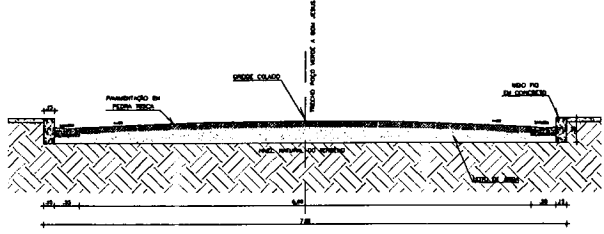
05 SEÇÃO TRANSVERSAL/DET. CONSTRUTIVO ESCALA - 1/25
