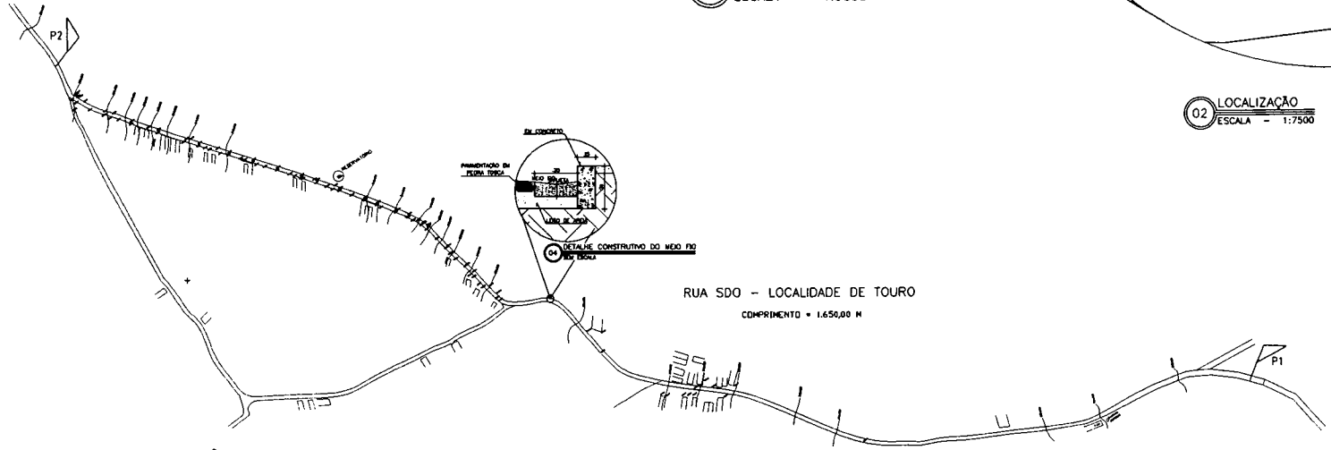
03 RUA SDO - LOC. DE TOURO ESCALA 1/2000
