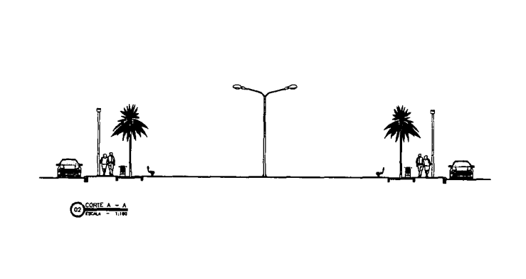
04 DET. DOS BANCOS SEM ESCALA
