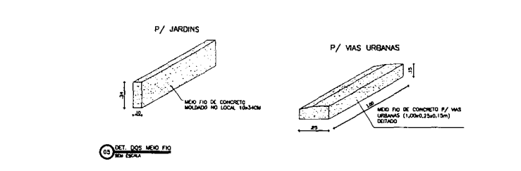
03 DET. DAS LINÉARIS SEM ESCALA
