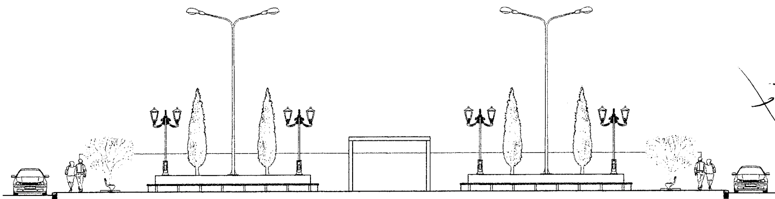
02 CORTA A-A ESCALA - 1:50
